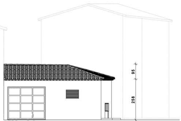
Façade Nord Est
