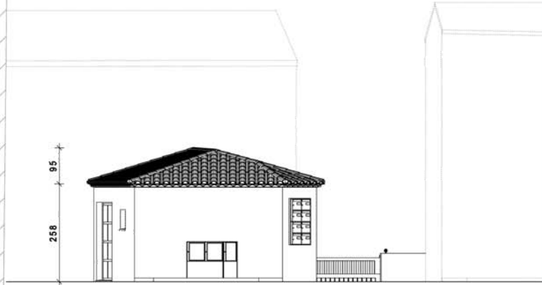
Façade Nord Ouest
